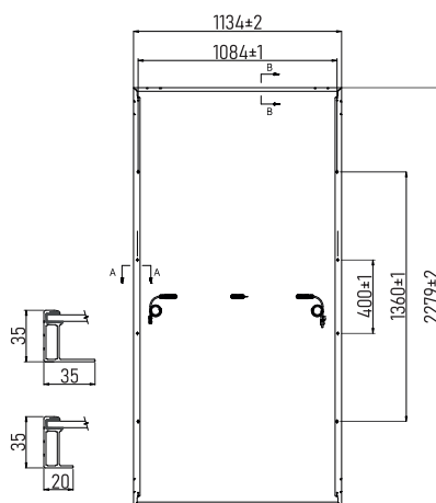
WYMIARY MODUŁU
