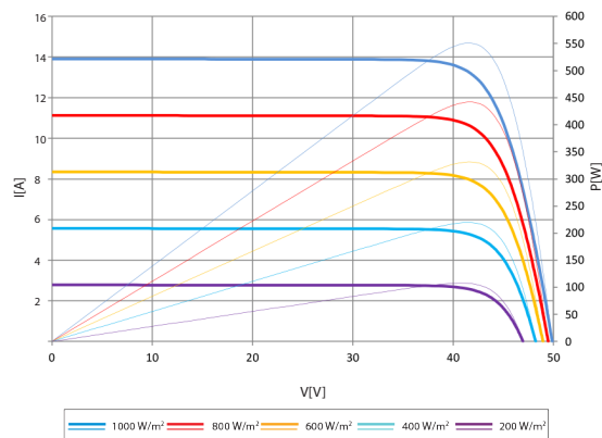
CHARAKTERYSTYKA PRĄDOWO-NAPIĘCIOWA
