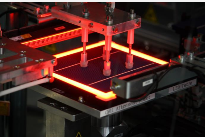
Linia technologiczna japońskiej firmy NPC
